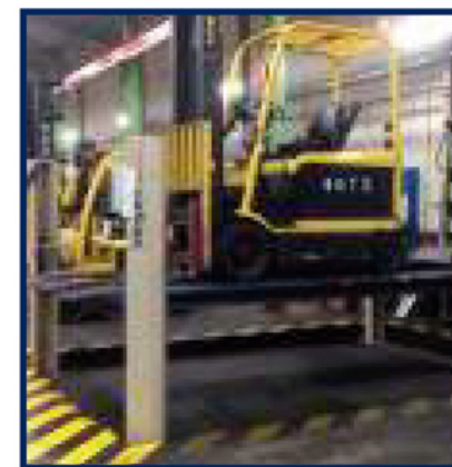
Elevador 4 Columnas Especial Carretillas 12.000 Kg
